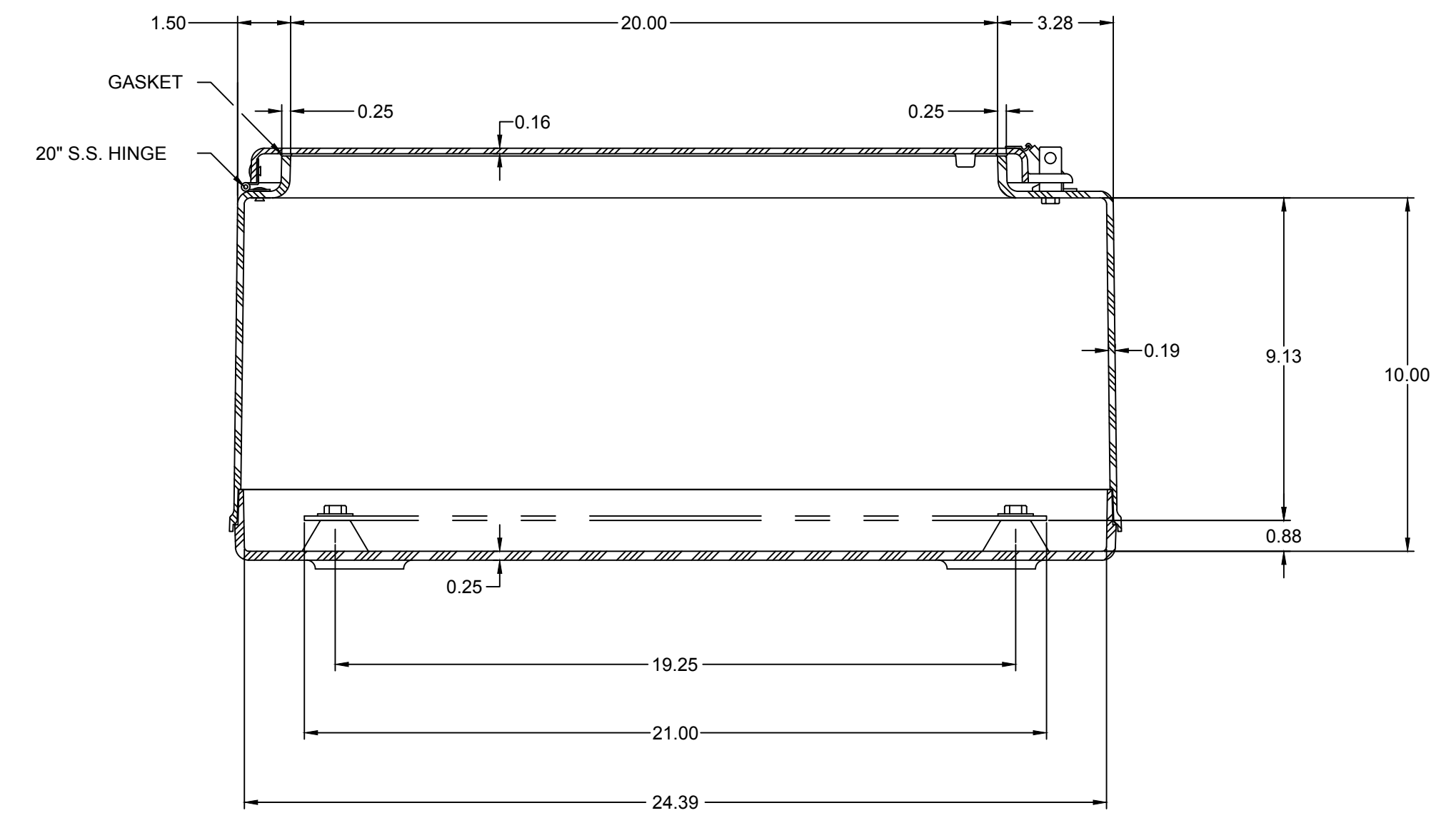
SECTION A-A
