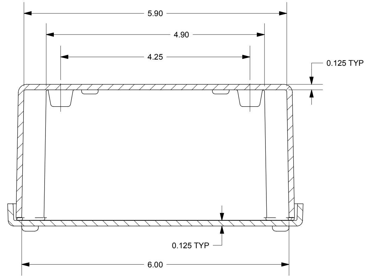
SECTION A-A
