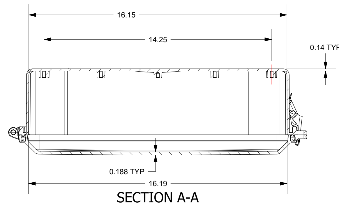
SECTION A-A
